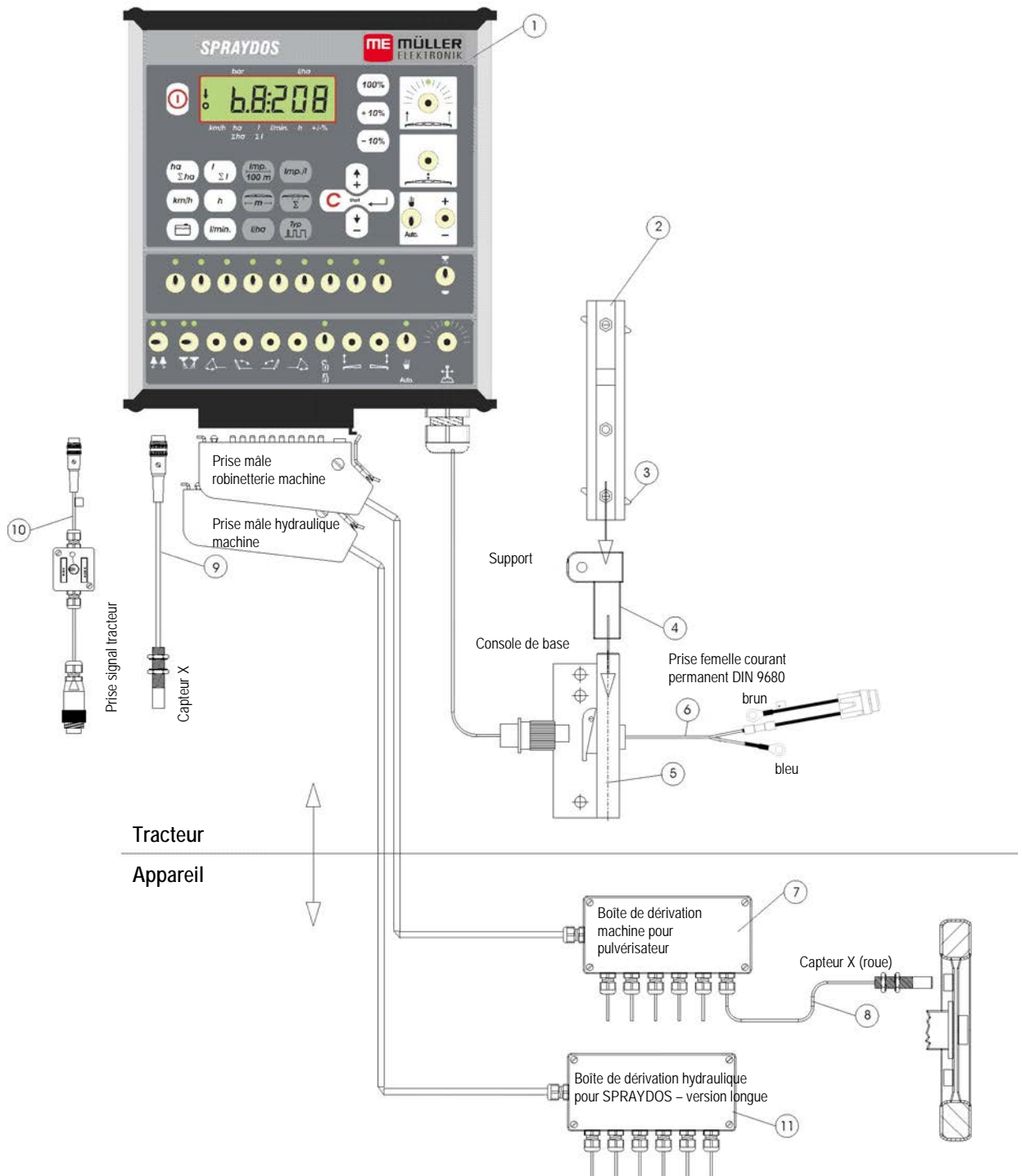
Fig. 4-1 Vue d'ensemble SPRAYDOS
